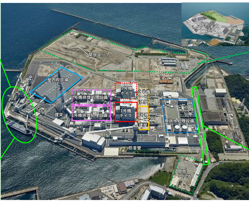
高波対策工事 開始 高波で海水が発電所内に侵入しないよう、コンクリート製の防波堤を建設します。
