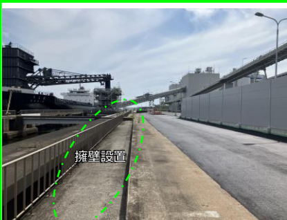
高波対策工事 開始 高波で海水が発電所内に侵入しないよう、コンクリート製の防波堤を建設します。
